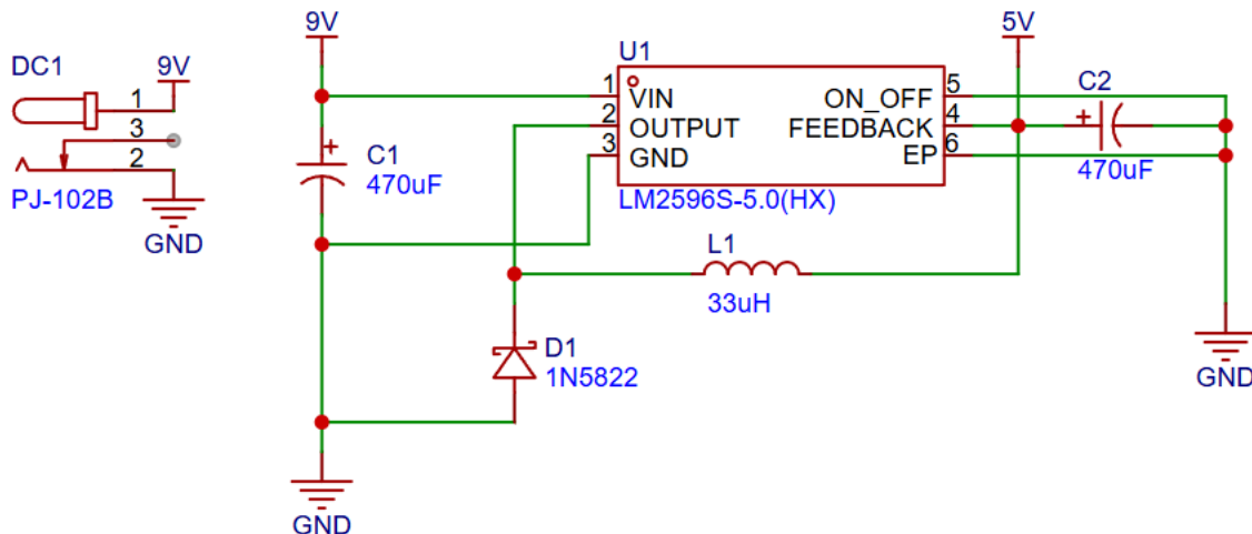
Hình 3.2: Sơ đồ nguyên lý mạch nguồn hạ áp từ 9 V xuống 5 V
