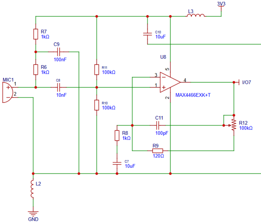
Hình 3.4: Sơ đồ nguyên lý mạch thu âm và tiền khuếch đại
