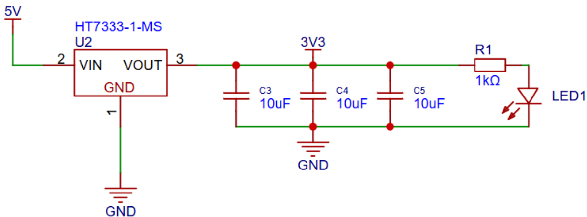
Hình 3.3: Sơ đồ nguyên lý mạch nguồn hạ áp từ 5 V xuống 3,3 V
